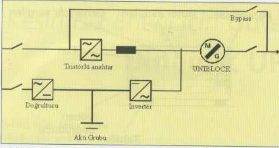
Şekil 4: PILLER UB-R Dinamik UPS'in tek hat şeması.
