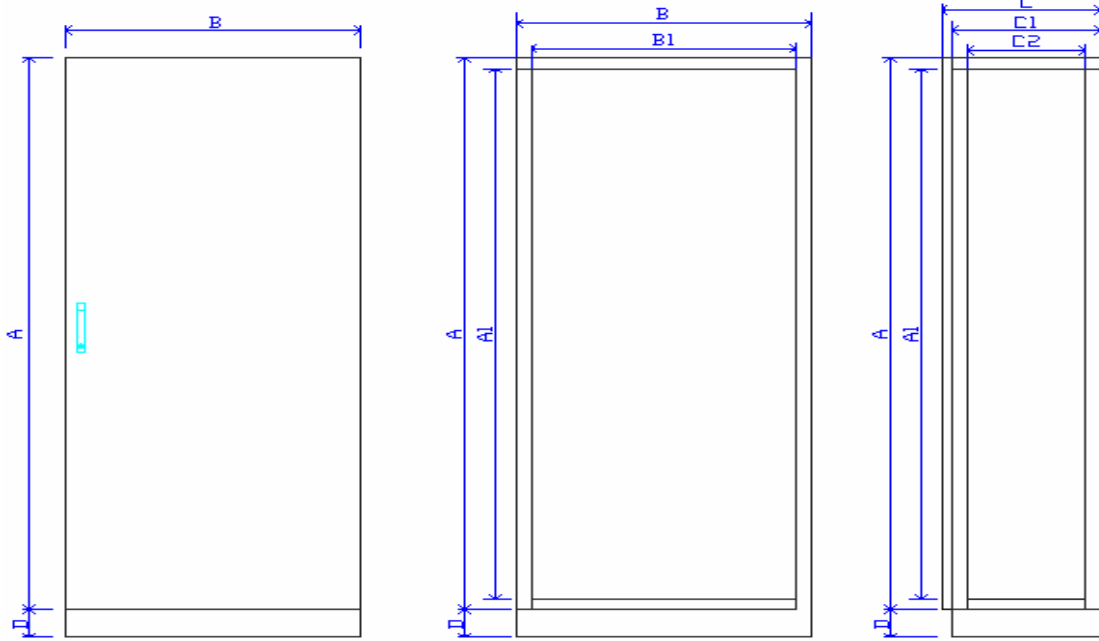
KAPI GÖRÜNÜŞÜ
